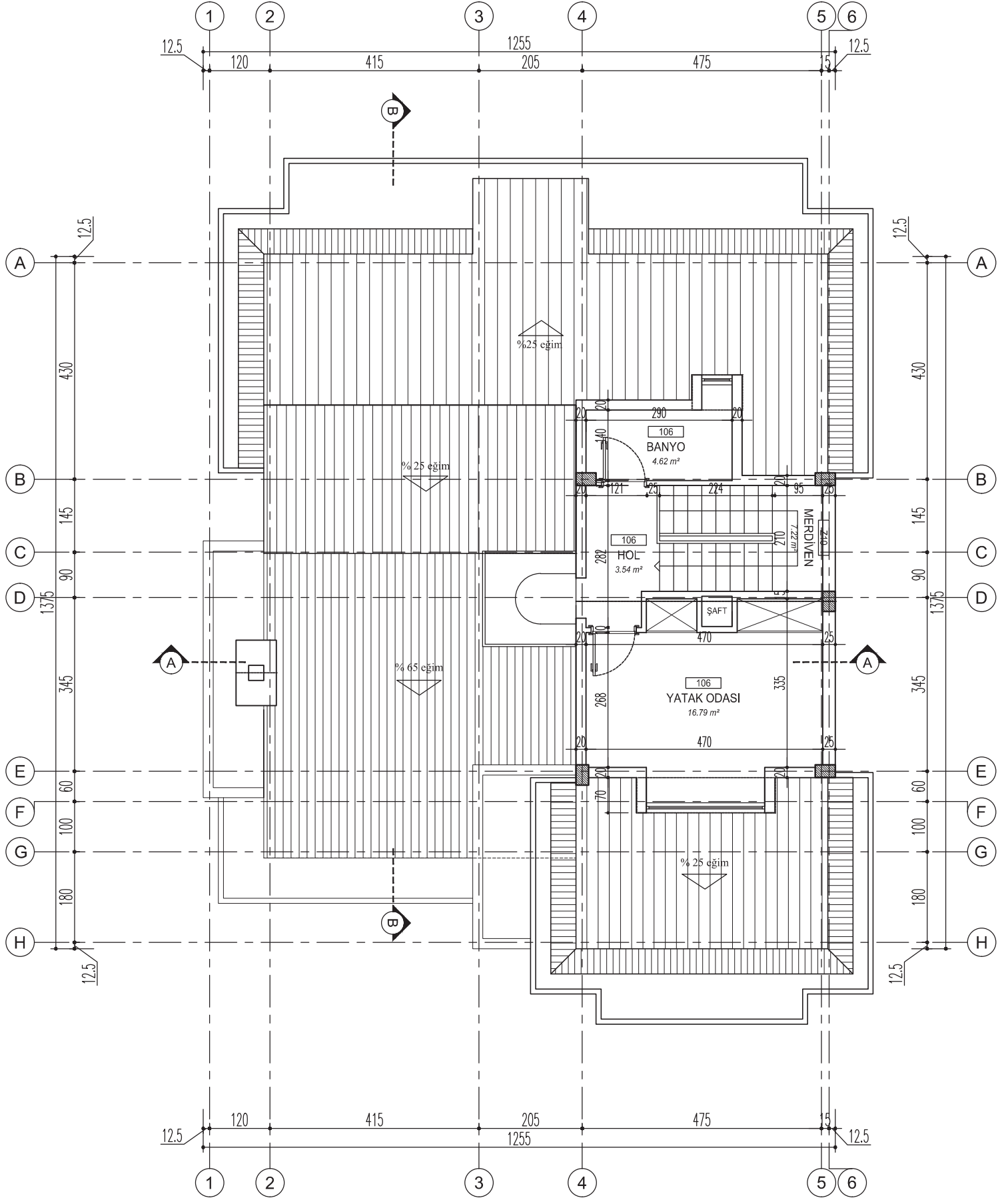
ÇATI KATI PLANI
